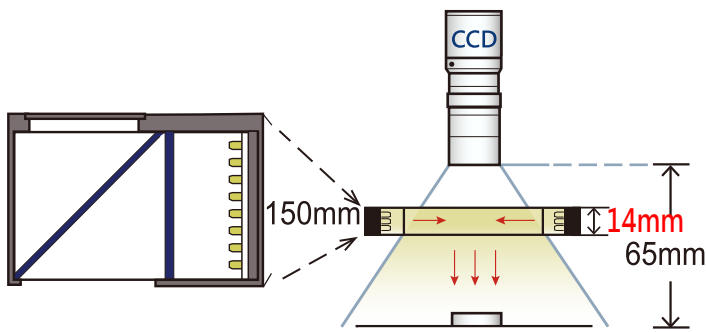
外同軸 CL-150140
